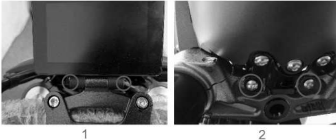
Ajuste de la altura del haz del faro
