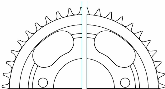
Piñón/Corona correcto
